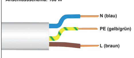
Anschlusschema: 150 W
