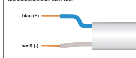
Anschlusschema: DALI Bus
