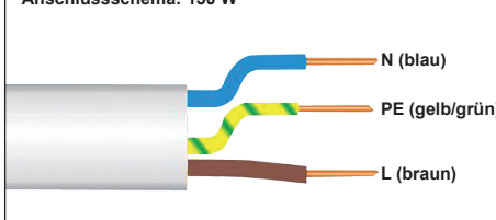
Anschlusschema: 150 W
